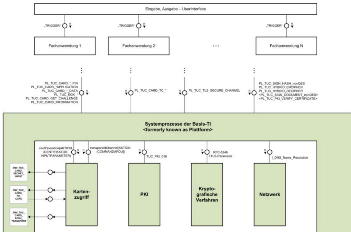
Abbildung 1: Systemprozesse der Basis-TI
