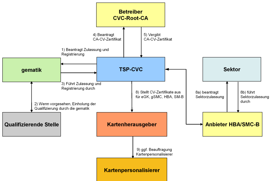
Abbildung 1: Beispielhafte Nachbarsysteme eines TSP-CVC
